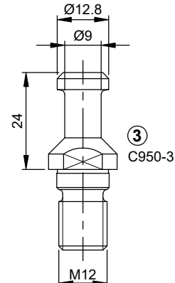
für Kegel SK 30: nach ISO - Norm (D1=46mm) CMS
