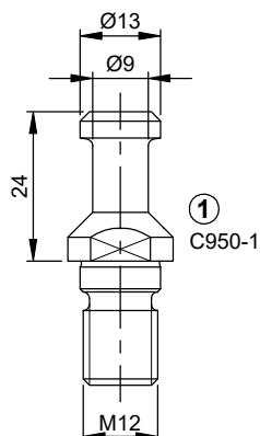
für Kegel SK 30: (DIN 69872) IMA, Maka, Reichenbacher, CMS, Weeke, Busellato, etc.
