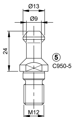
für Kegel SK 30: Alberti, Masterwood (Colombo Motoren)
