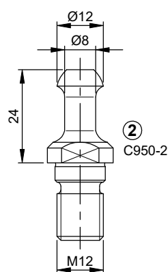
für Kegel SK 30: Biesse ab Baujahr 9/92, Masterwood (HSD-Motoren)
