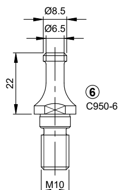
für Kegel SK 30 mit Zahnkranz: Morbideilli, SCM
