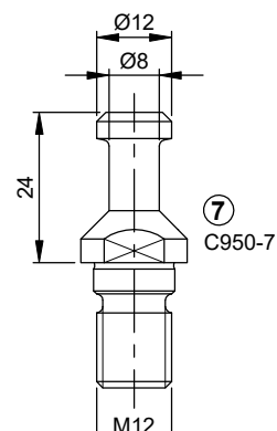
für Kegel SK 30: Biesse bis Baujahr 9/92
