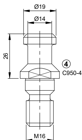
für Kegel SK 40: (DIN 69872) IMA, Maka, Reichenbacher, Stegherr, etc.
